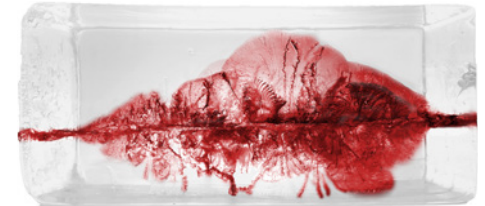
→ Simulierte Wundhöhle in ballistischer Gelatine: Kal. .30-06 auf 100 m
